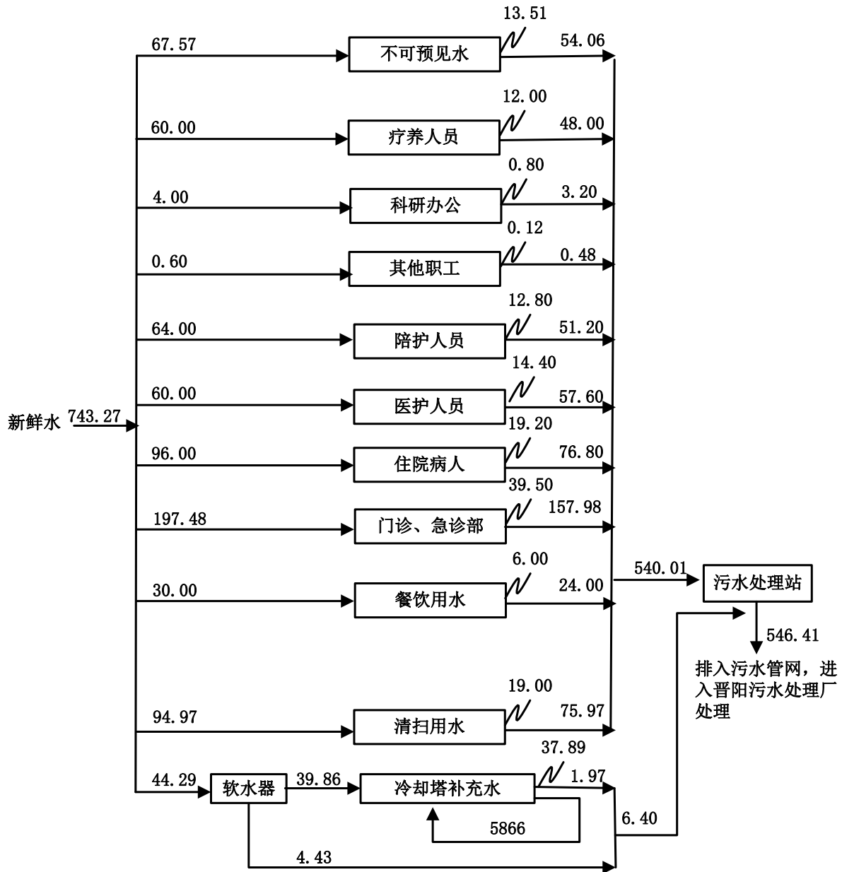
图 3.3-4 全院水平衡图（采暖期） 单位：m³/d
