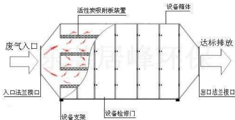
图 6.2-2 活性炭吸附工艺流程图
